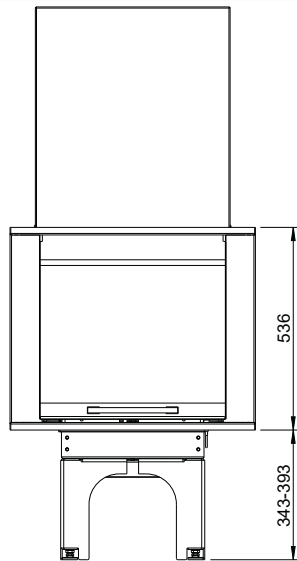
Blendrahmen am KALA QS/PS/US mit Set Blenden 4-teilig (oben + unten + seitlich) / M1:20
