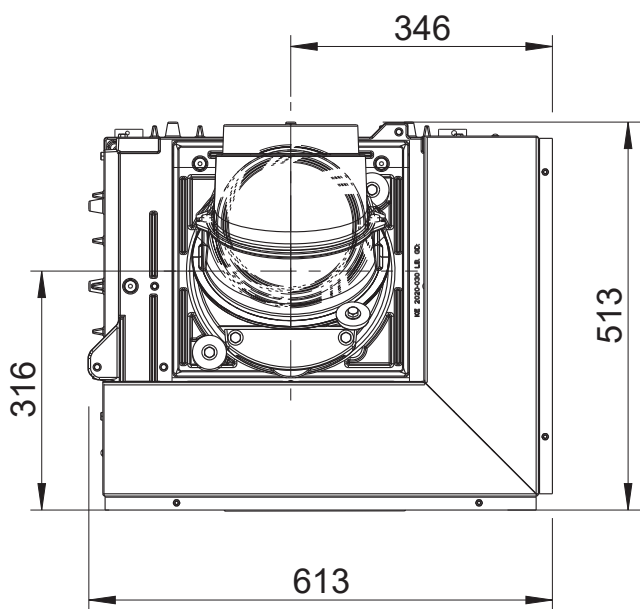
KALA H ES 55 R Draufsicht / M1:10
