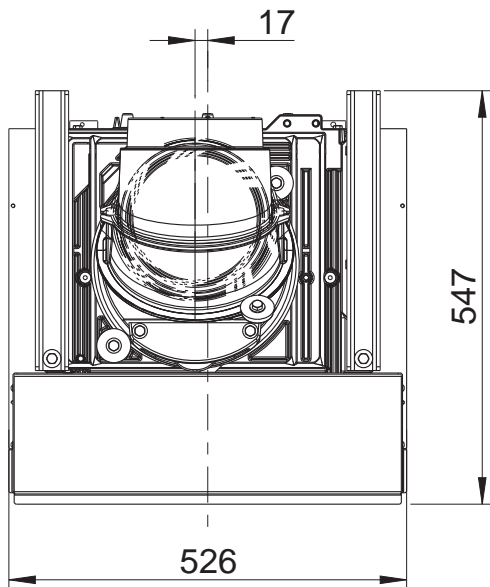
KALA QS Draufsicht / M1:10
