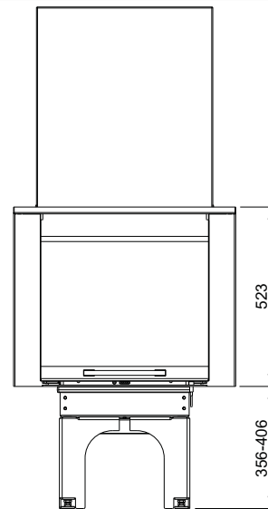
Blendrahmen am KALA QS/PS/US mit Set Blenden 3-teilig (oben + seitlich) / M1:20
