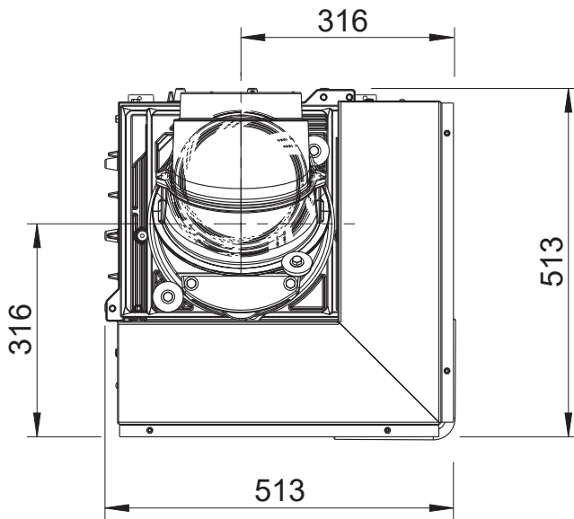
KALA H ES 45 Draufsicht / M1:10
