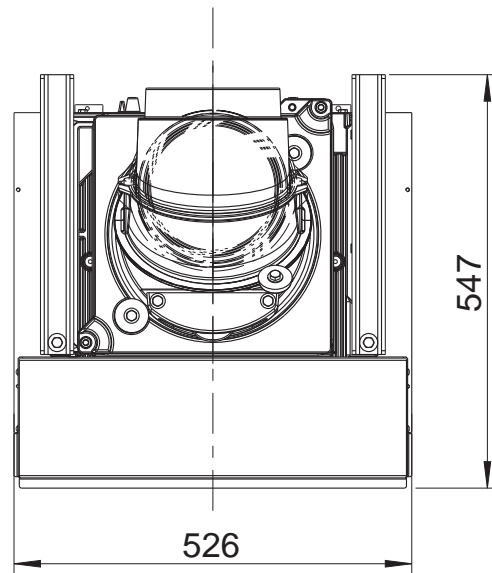
KALA QS mit Speicheraufsatz Draufsicht / M1:10
