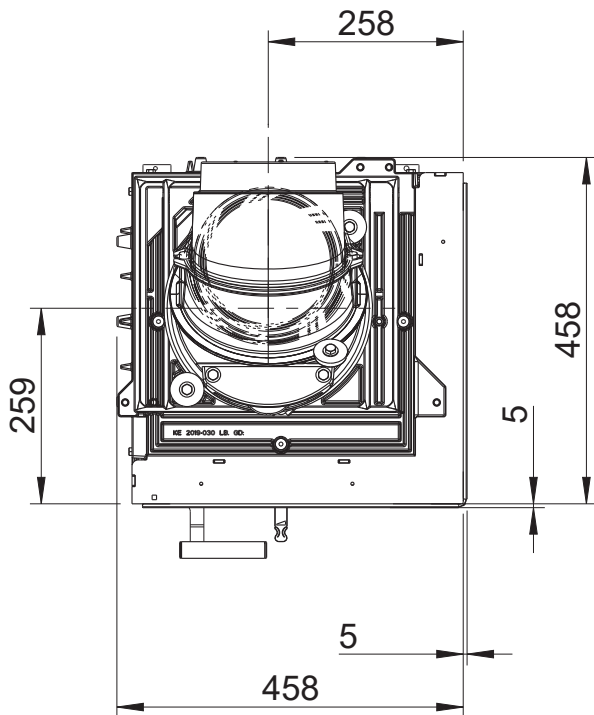
KALA S ES 45 R Draufsicht / M1:10
