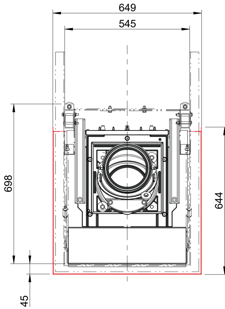
KALA US mit Blenden und Traggestell Draufsicht / M1:10
