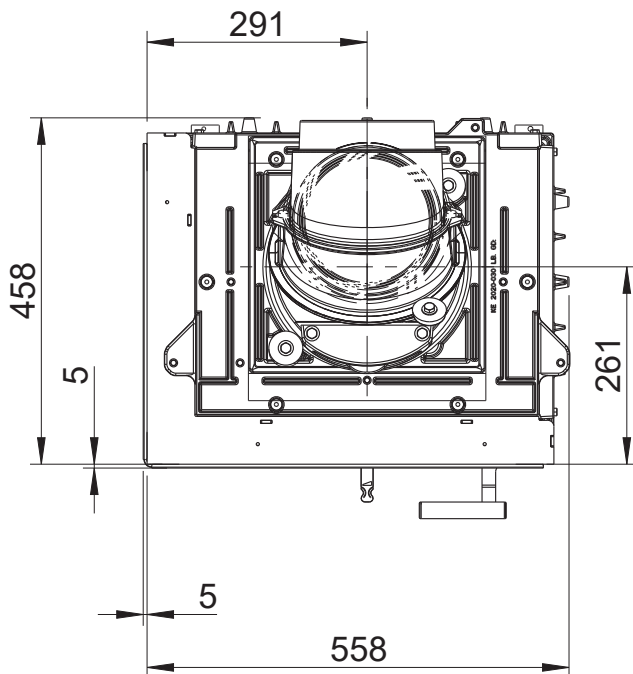
KALA S ES 55 L Draufsicht / M1:10
