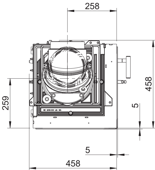
KALA S ES 45 L Draufsicht / M1:10
