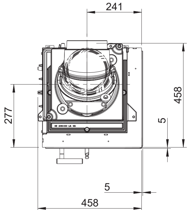
KALA S ES 45 R mit Speicheraufsatz Draufsicht / M1:10
